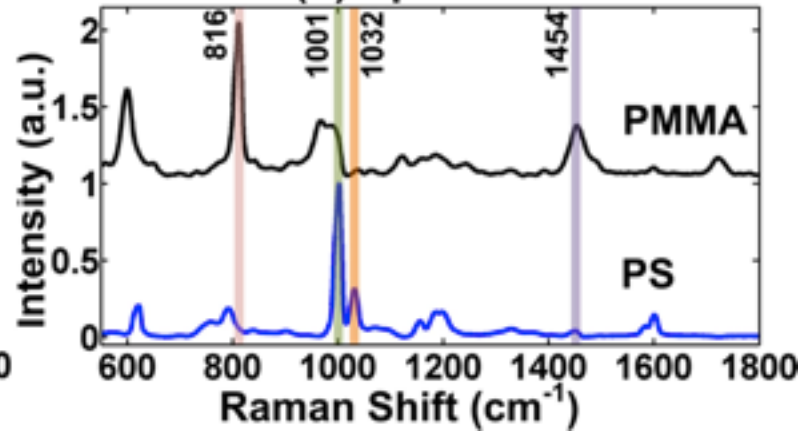
(d) Spectra
